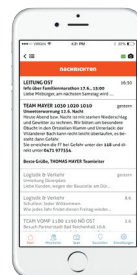
Sicheres Messaging
